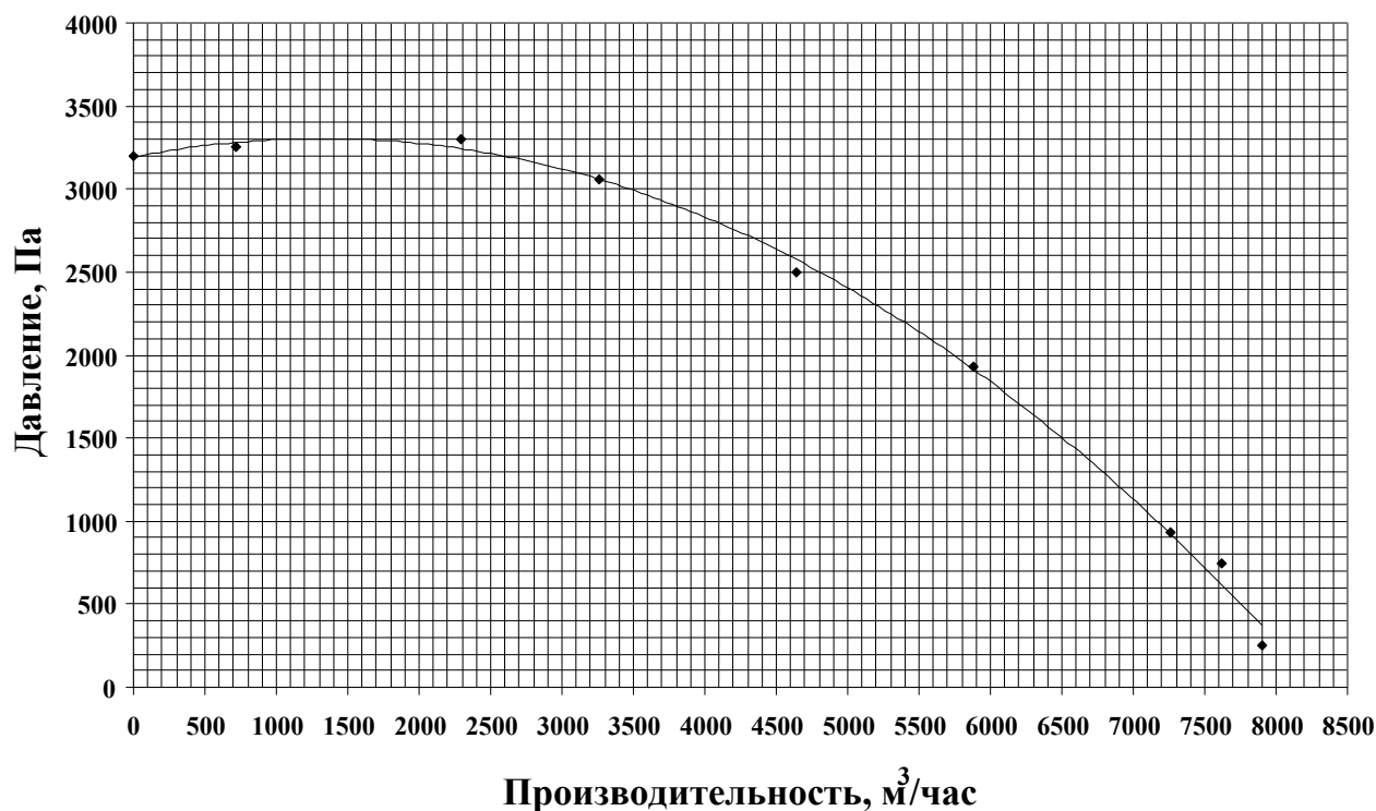
Характеристика МВФ-6000ДП (Статическое давление)
